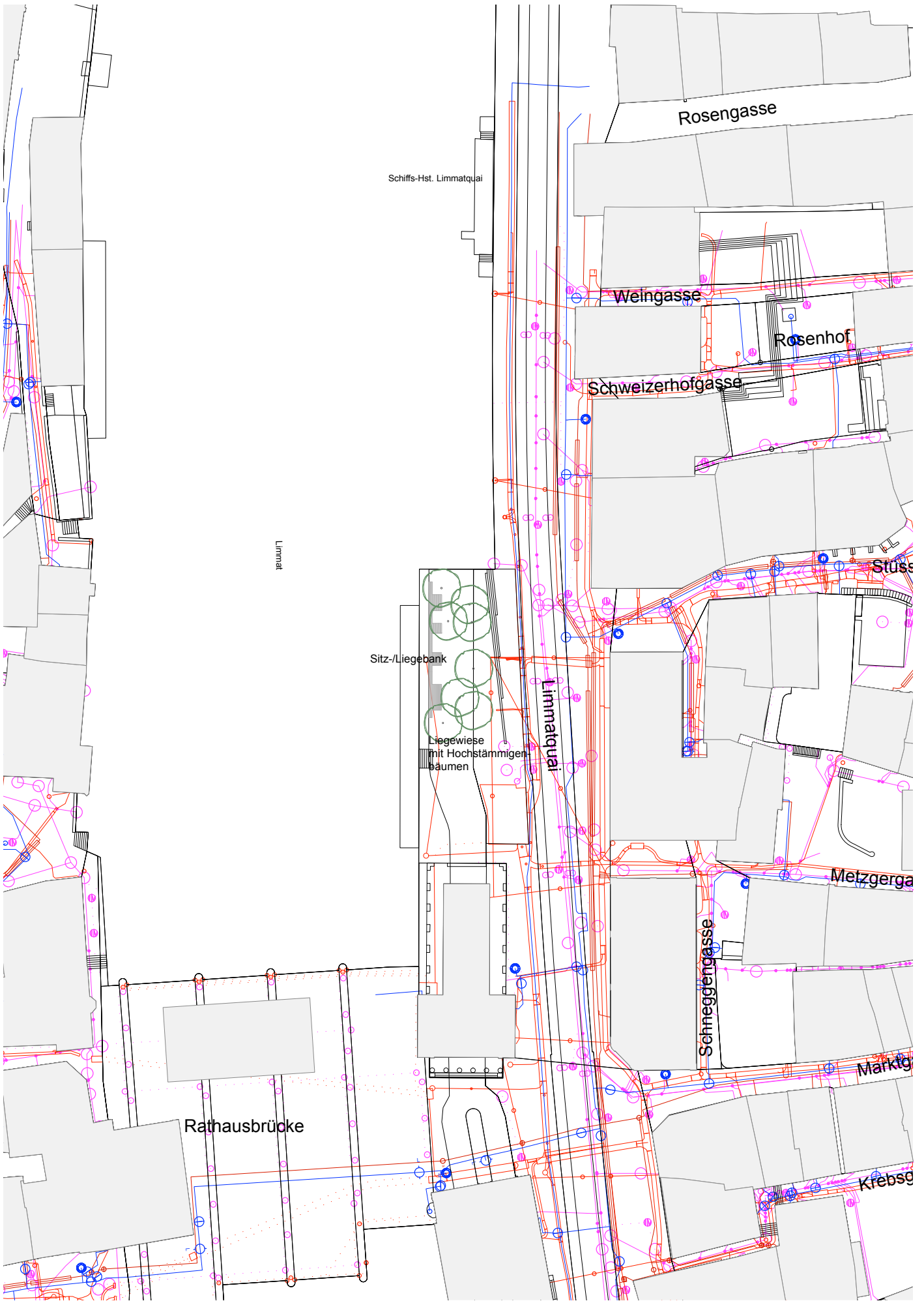
Werkleitungen
