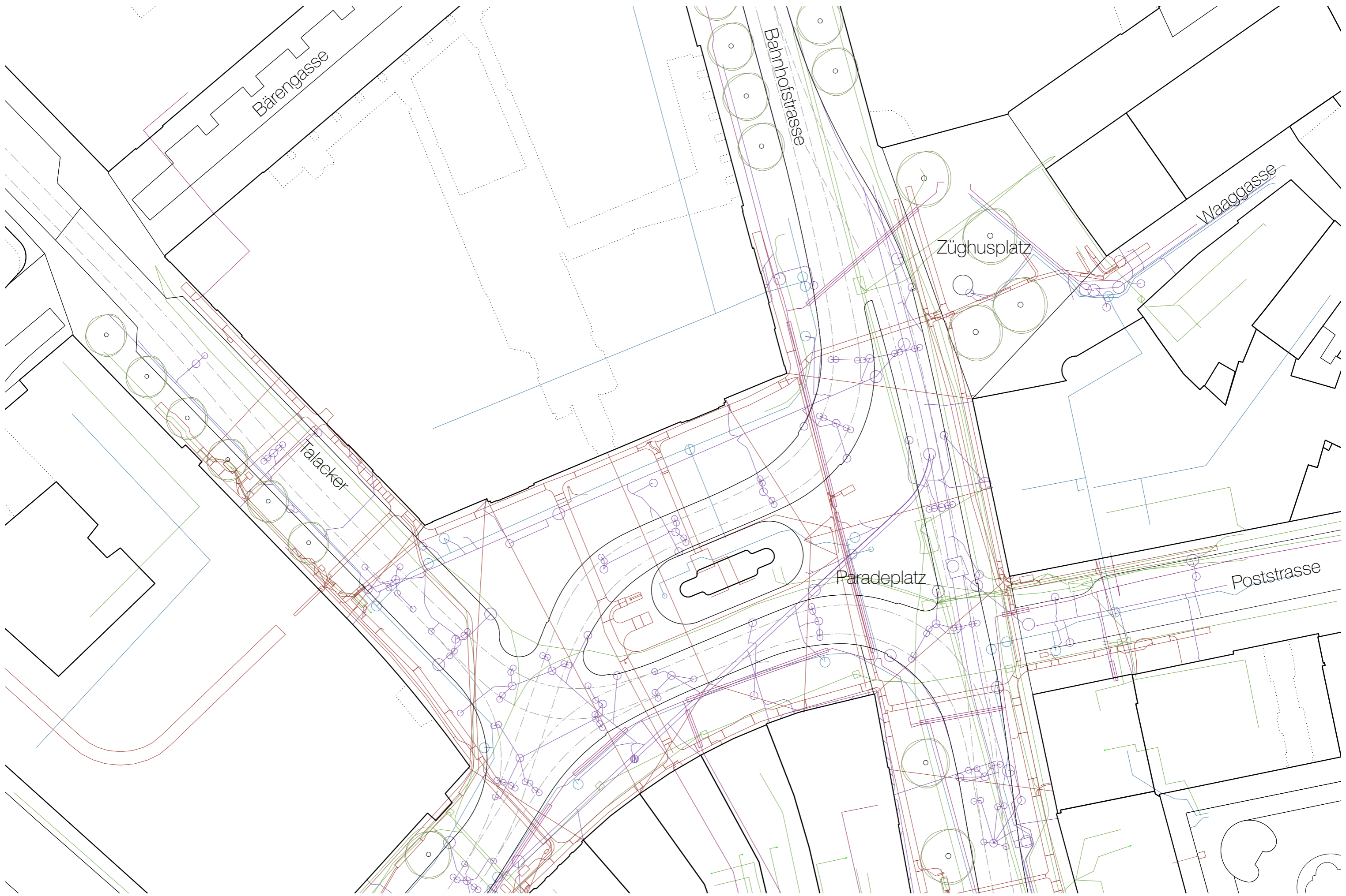
Situation / Werkleitungen Heute 1:500
